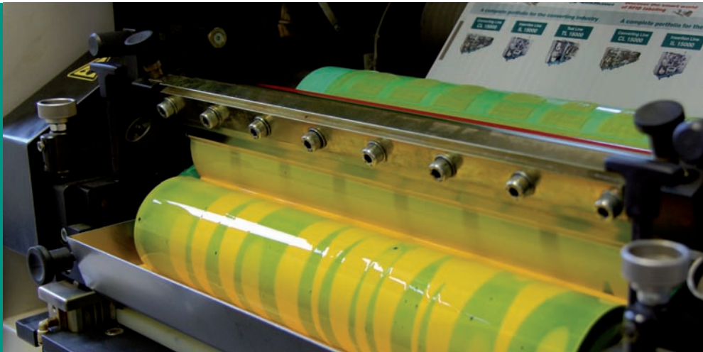
Druckwerk
