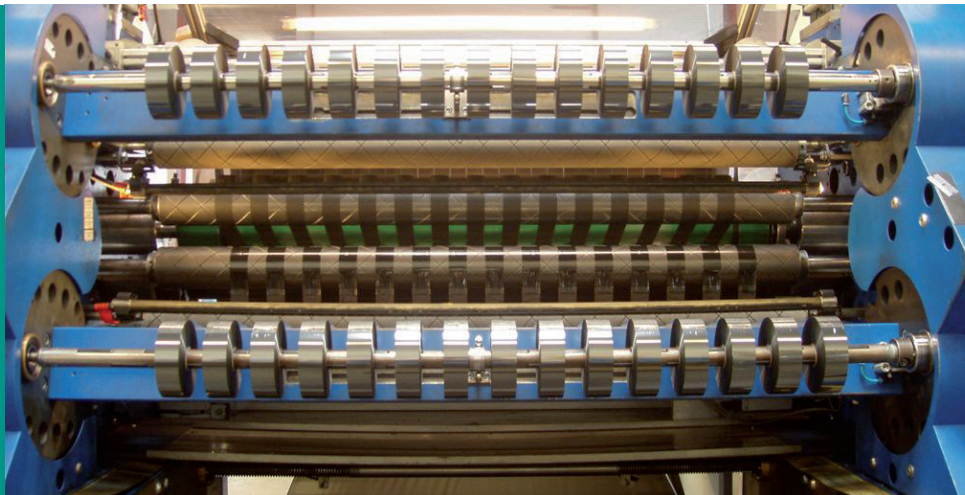
Schneidemaschine
