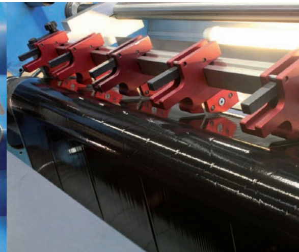
Längsschneider
